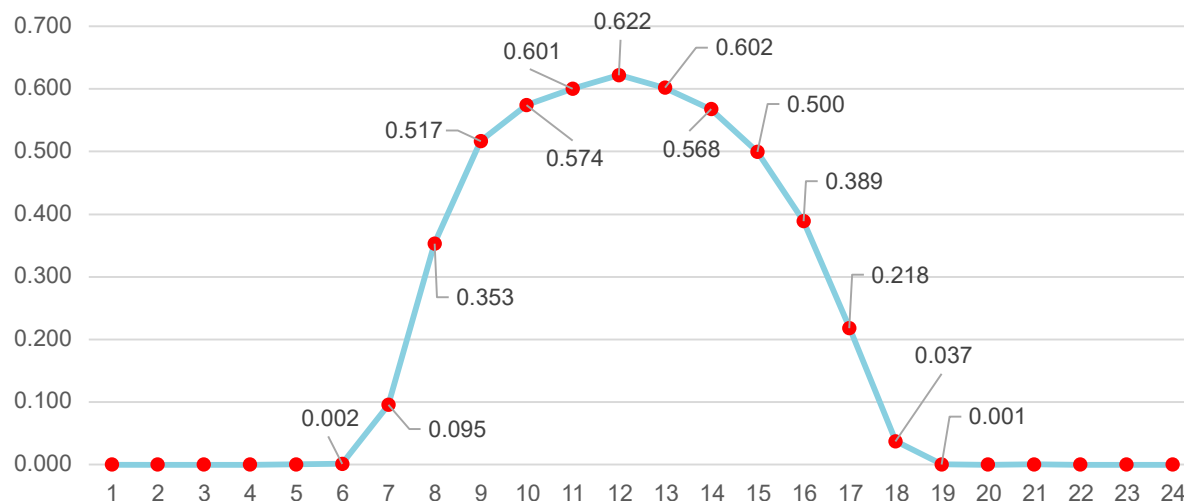
Gráfica 14 - Curva típica de generación solar en Honduras [p. u.], Base P.U.= 509.51 MW
