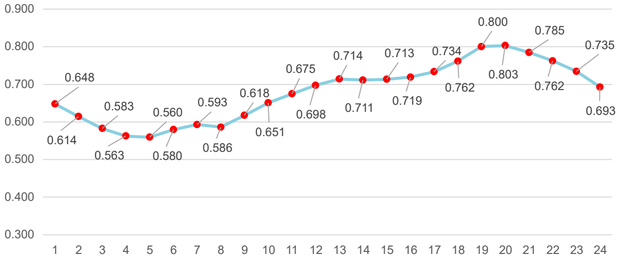
Gráfica 16 - Curva típica de generación fósil (búnker) zona norte de Honduras [p. u.]
