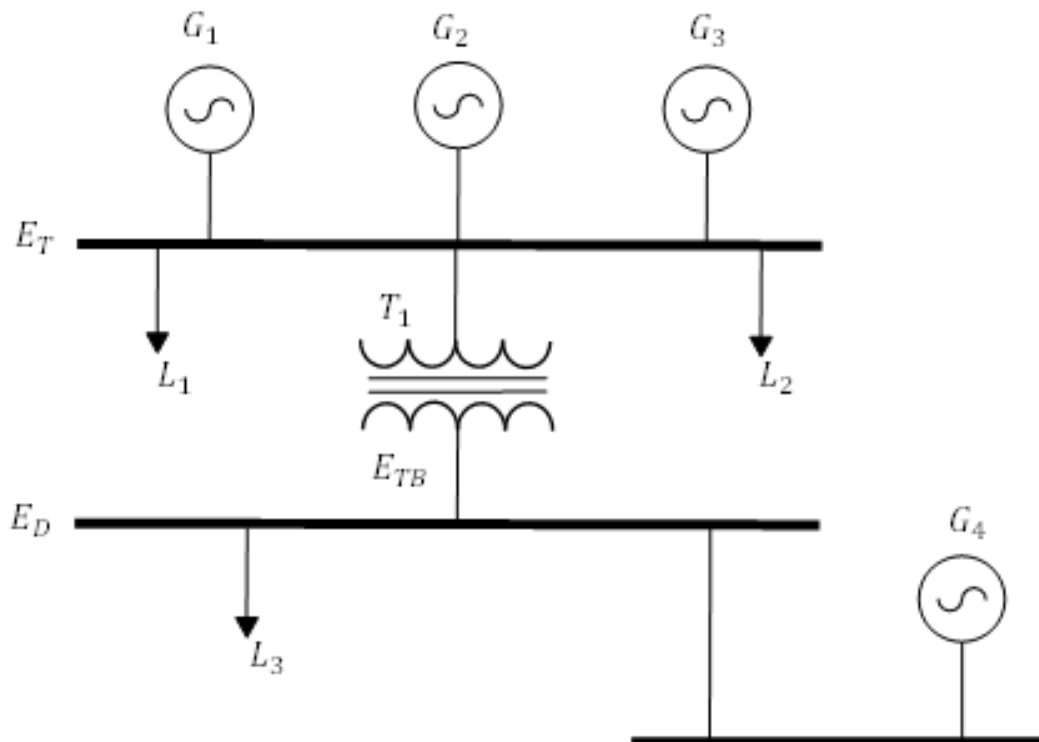
Ilustración 20 – Diagrama para cálculo de pérdidas eléctricas
