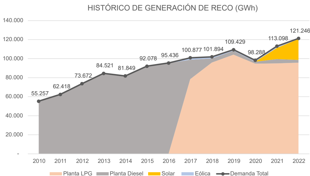
Gráfica 81 - Histórico de generación de RECO 2015-2022[GWh]
