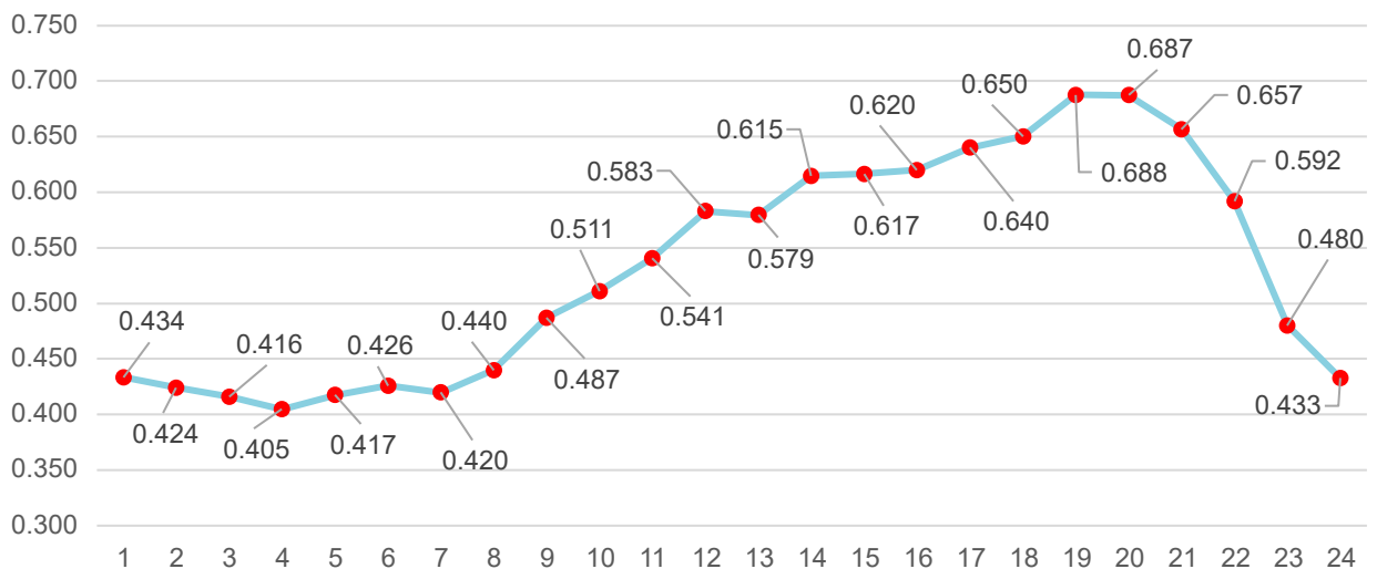
Gráfica 17 - Curva de generación típica de la central hidroeléctrica Francisco Morazán [p. u.]
