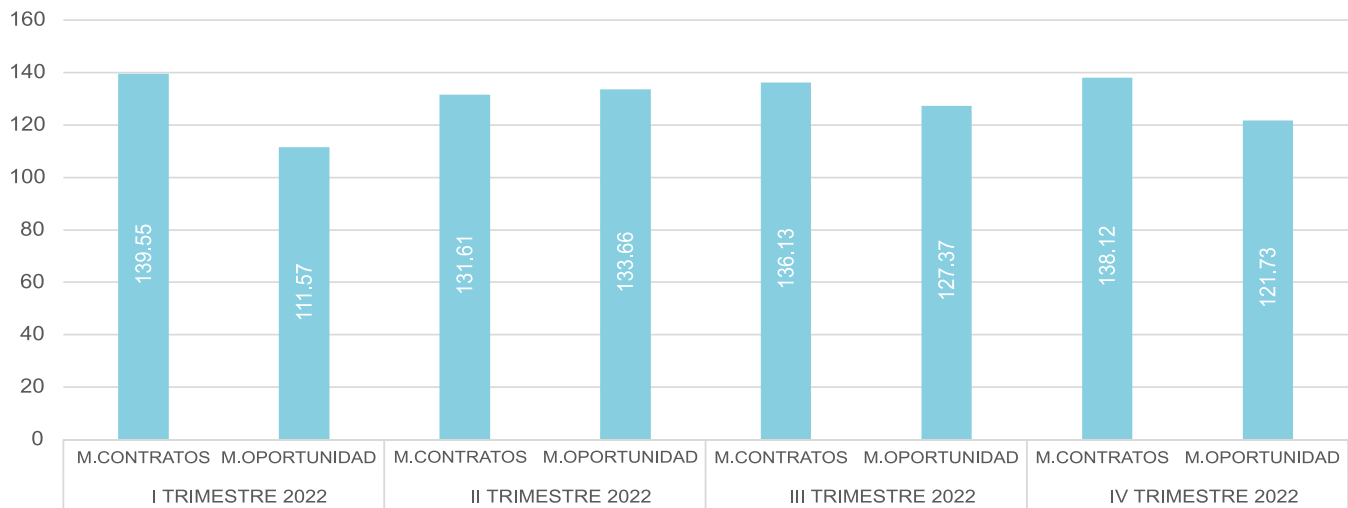
Gráfica 70 - Costos bases de Generación por tipo de mercado por trimestre del 2022
