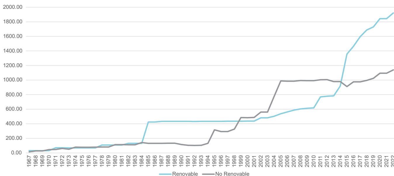
Gráfica 4 - Histórico de potencia eléctrica instalada por tipo de tecnología [MW] 1967-2022
