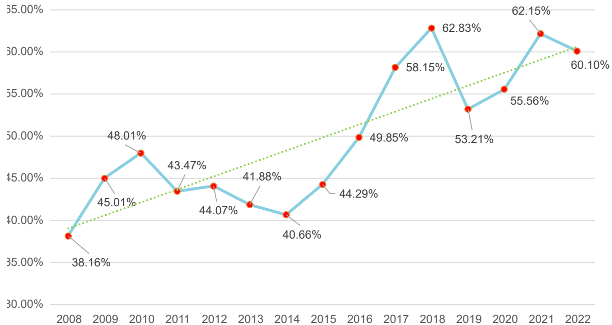
Gráfica 11 - Porcentaje histórico de renovabilidad en Honduras - Energía generada 2008-2022
