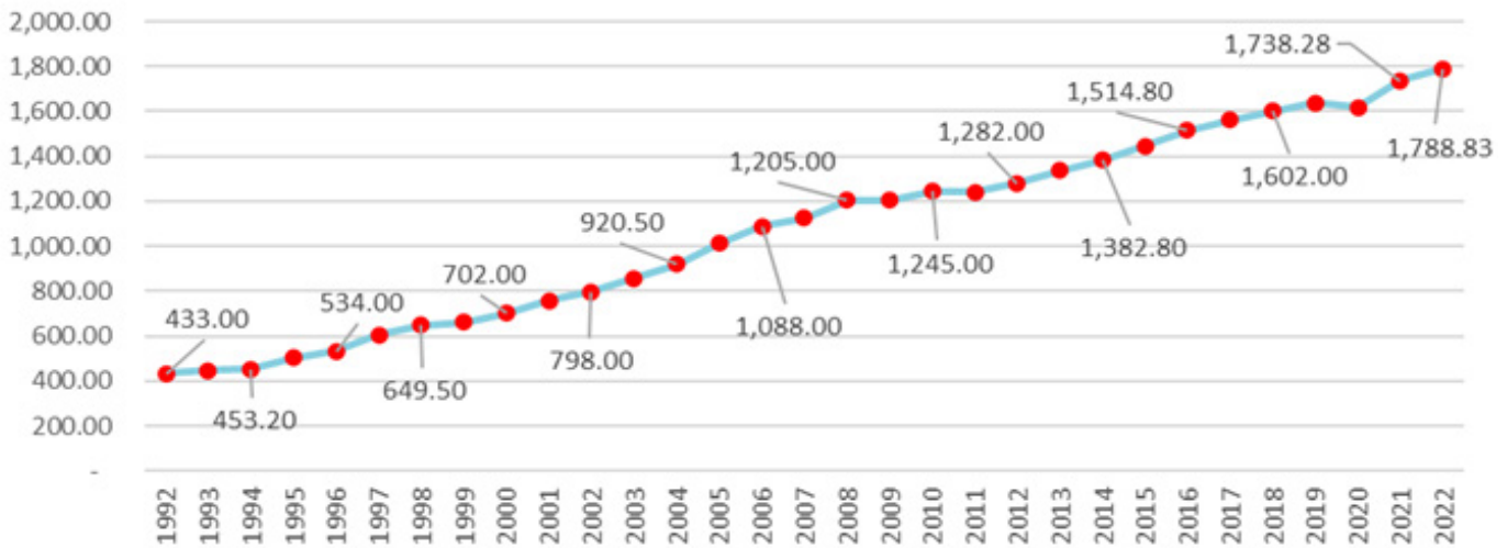
Gráfica 41 – Histórico de demanda máxima anual [MW] en Honduras 1992-2022
