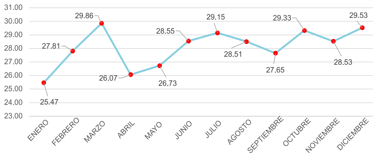
Gráfica 26 - Curva de generación anual de una planta geotérmica en Honduras [GWh]
