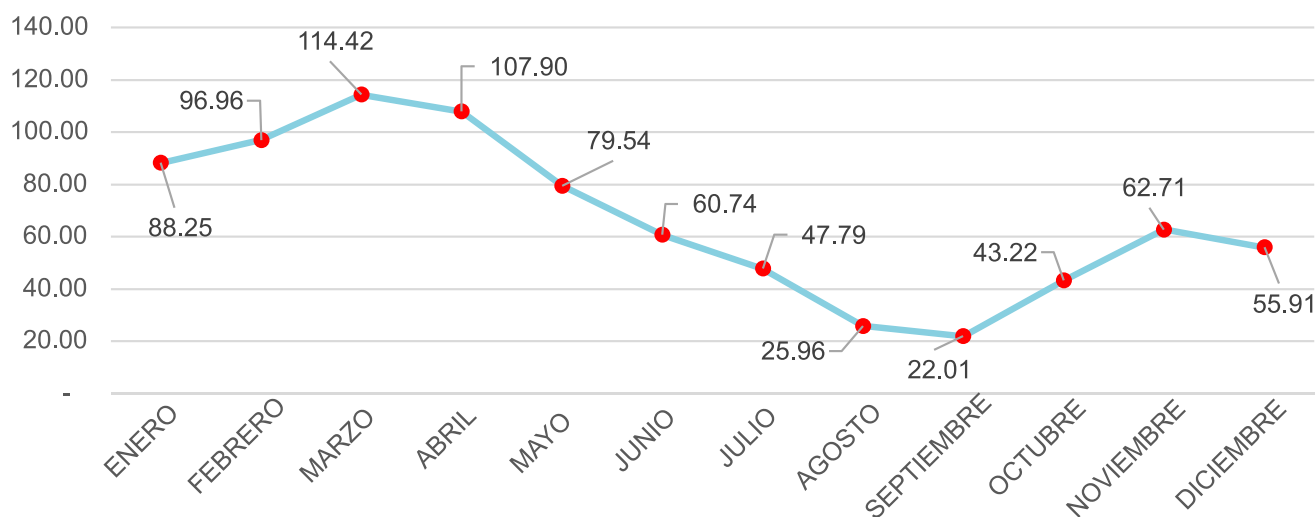
Gráfica 25 - Curva de generación anual para plantas de biomasa [GWh]
