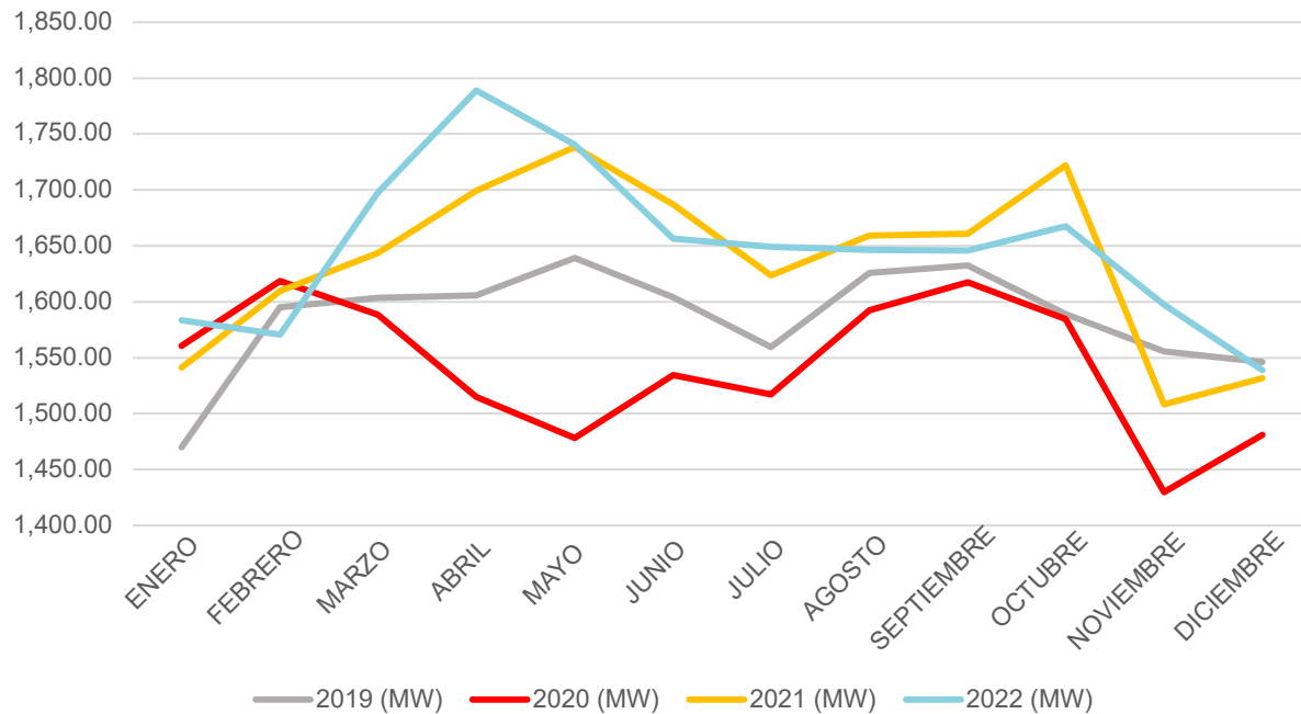
Gráfica 98 - Comparación de demanda máxima mensual 2019, 2020, 2021, 2022 [MW]
