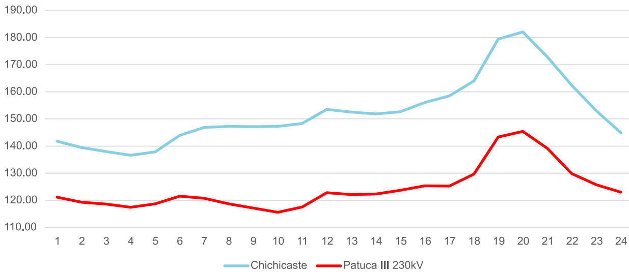
Gráfica 53 - Costo marginal promedio del nodo más caro y el nodo más barato del SIN [USD/MWh]
