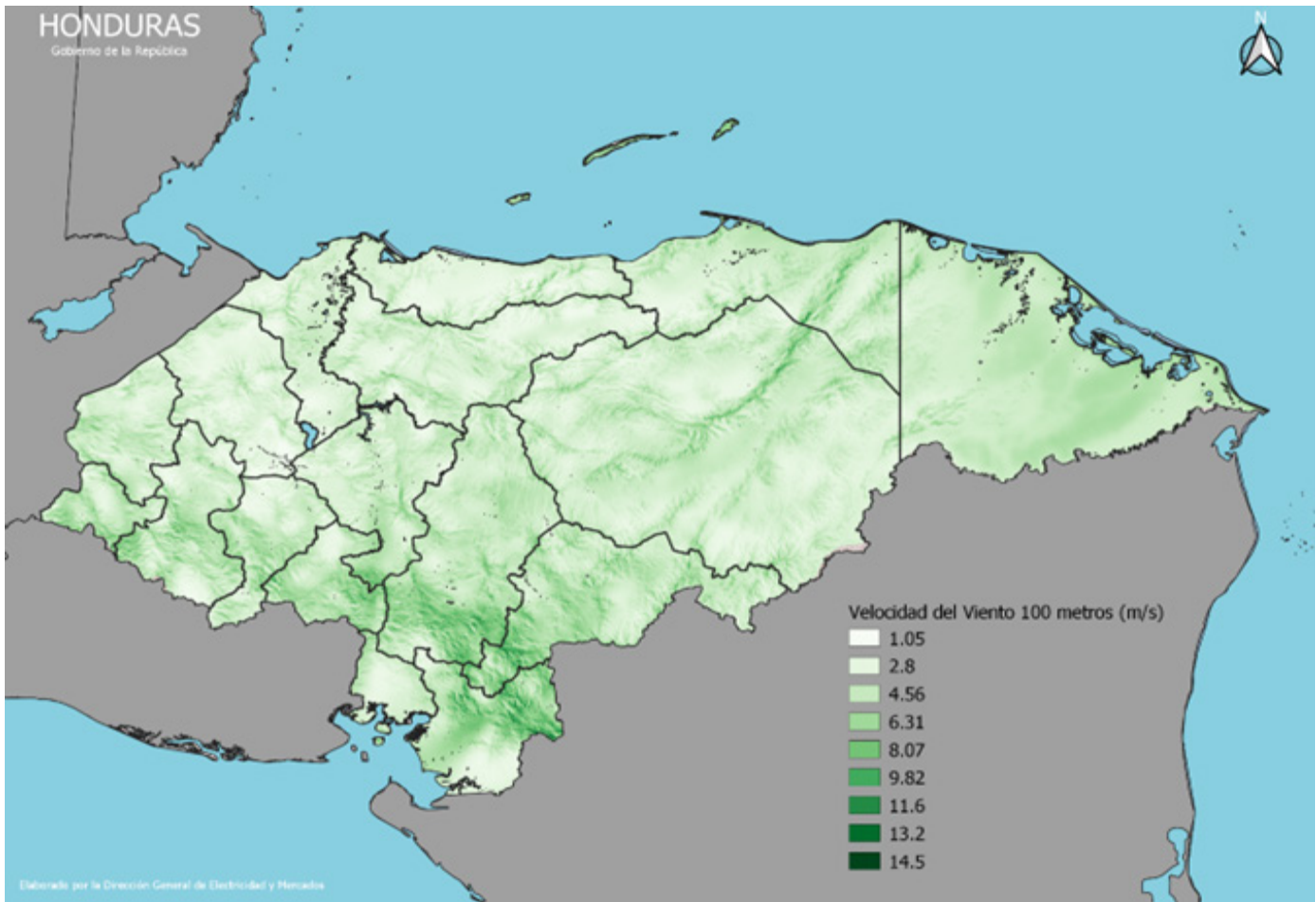
Ilustración 9 - Mapa de potencial eólico de Honduras
