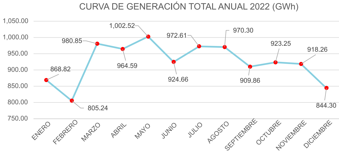
Gráfica 27 - Energía total generada mensual en el año 2022 en Honduras [GWh] Fuente: Centro Nacional de Despacho (CND)
