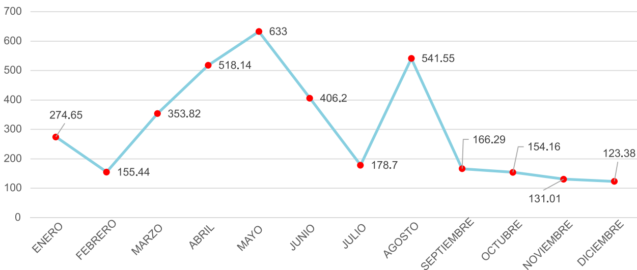
Gráfica 54 - Costo marginal máximo mensual del nodo Santa Fe 138 kV [USD/MWh]
