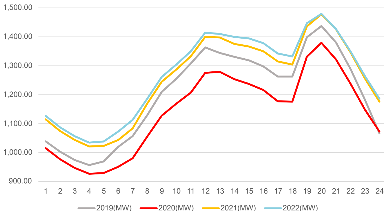
Gráfica 96 - Comparación de demanda promedio 2019, 2020, 2021, 2022 [MW]
