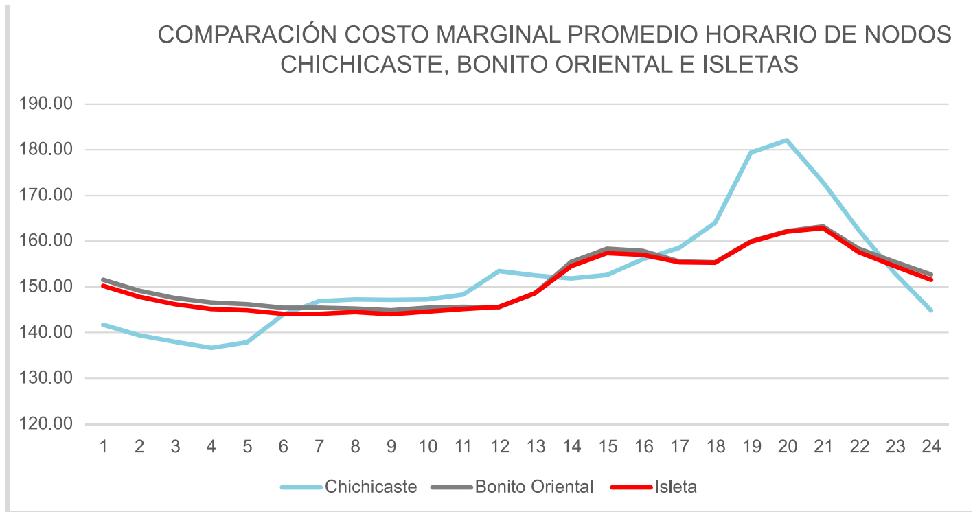
Gráfica 57 - Comparación entre los nodos con los costos marginales promedio más altos [USD/MWh]
