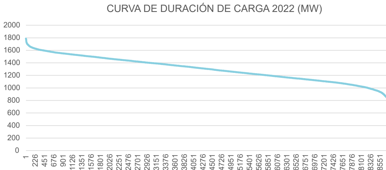
Gráfica 38 - Curva de máxima duración de carga 2022 [MW]
