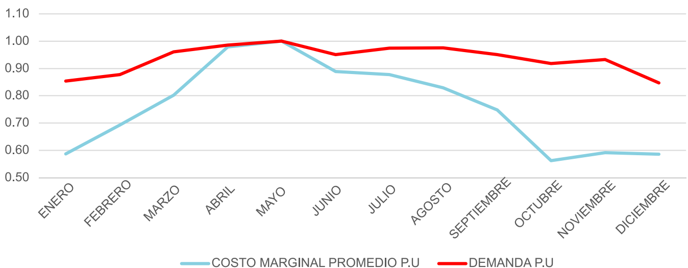
Gráfica 56 - Comparación de tendencias P.U. entre costo marginal mensual promedio y demanda de energía
