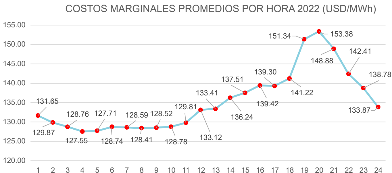
Gráfica 51 - Costo marginal promedio por hora 2022 [USD/MWh]
