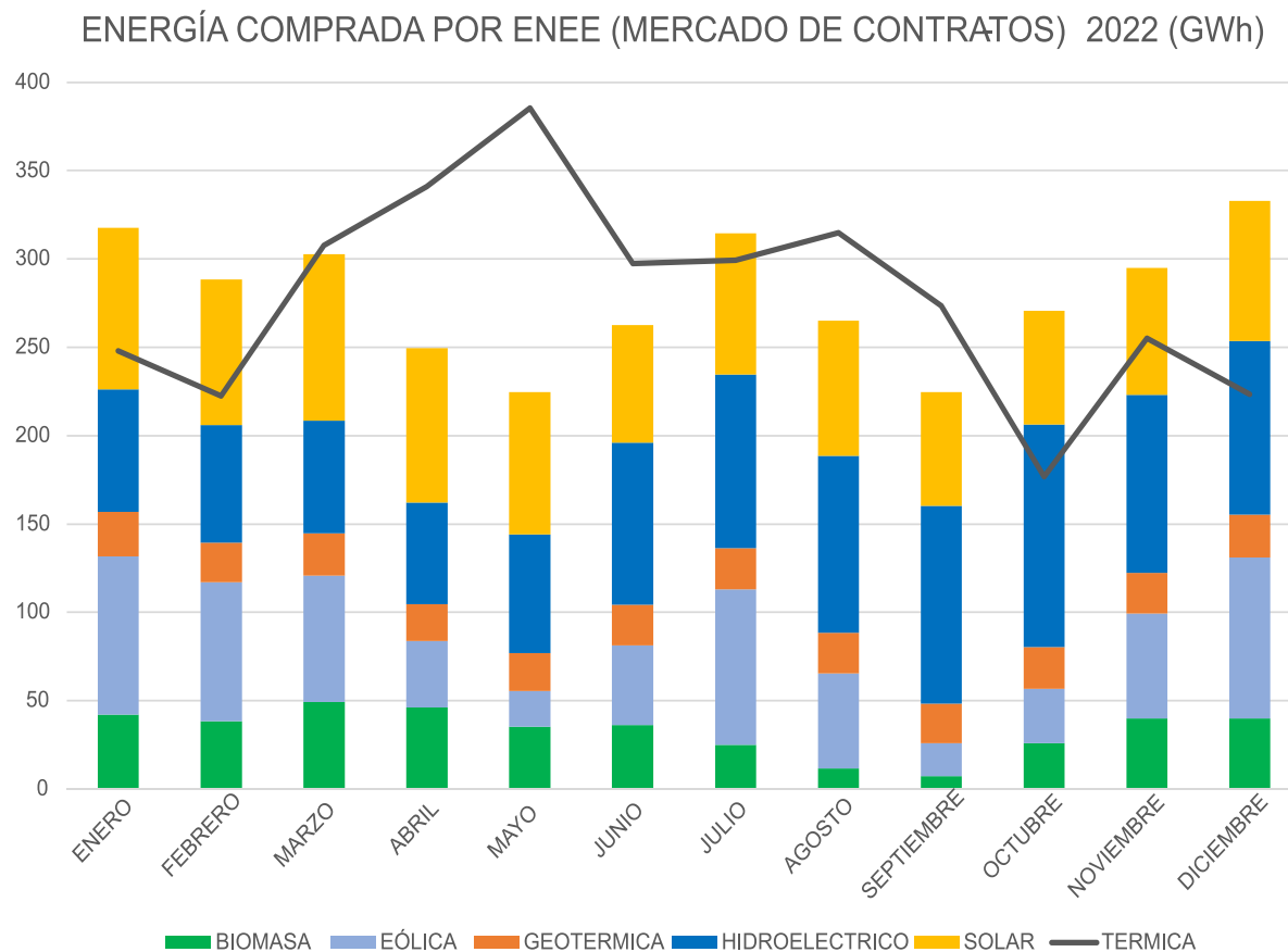
Gráfica 28 - Energía mensual comprada por ENEE distribución 2022 [GWh]
