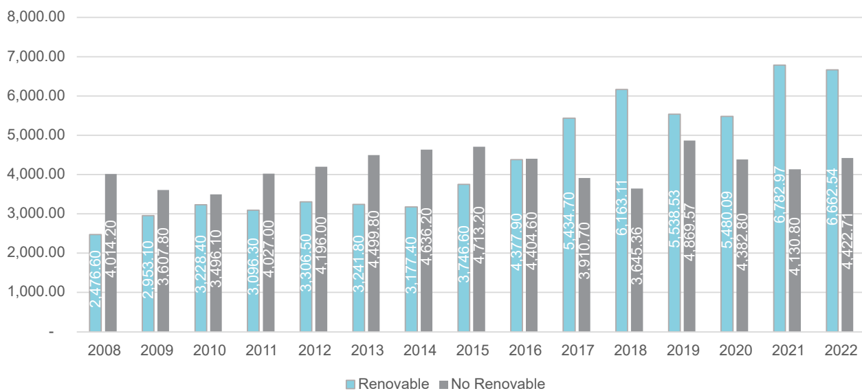
Gráfica 12 - Generación histórica (GWh) por tipo de tecnología
