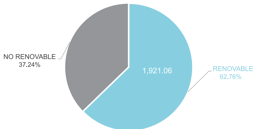
Gráfica 1 - Potencia eléctrica instalada en Honduras por tipo de fuente
