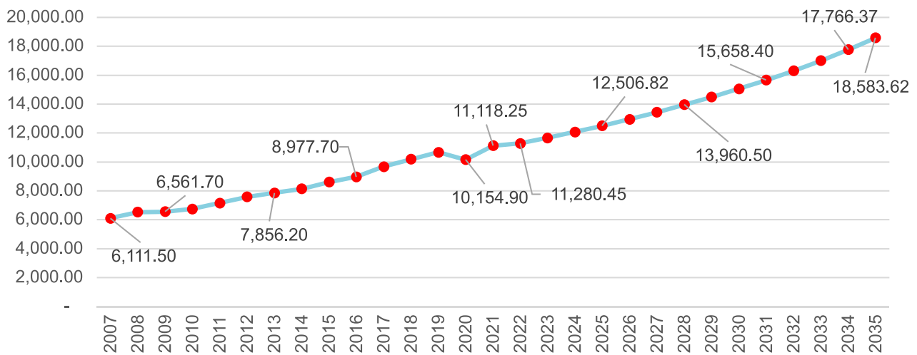
Gráfica 42 – Proyección de demanda [MW] para Honduras 2022-2035
