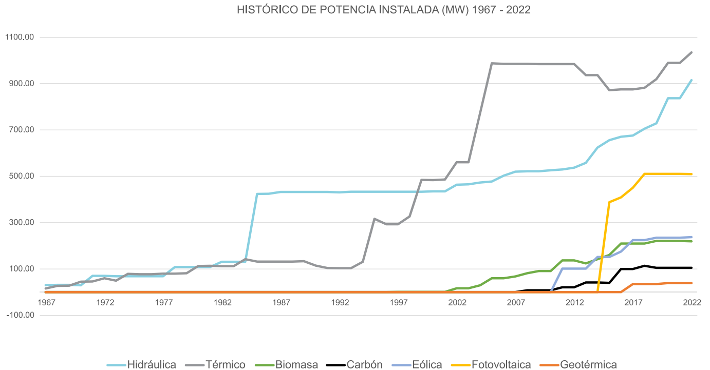
Gráfica 3 - Histórico de potencia instalada [MW] 1967-2022
