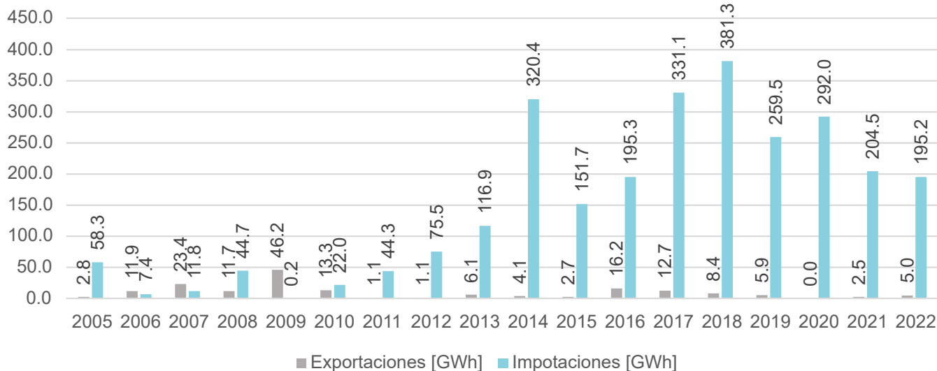
Gráfica 78 - Histórico de compras y ventas en el de energía eléctrica en el MER [GWh]
