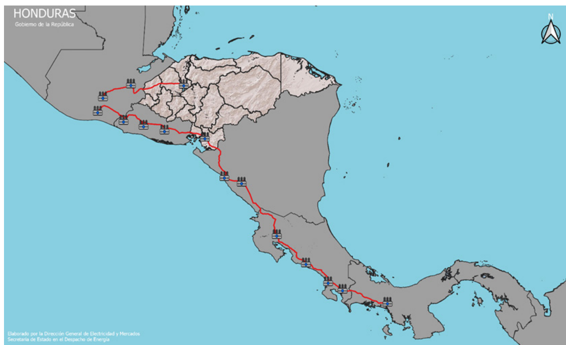
Ilustración 21 - Mapa de la línea de transmisión SIEPAC
