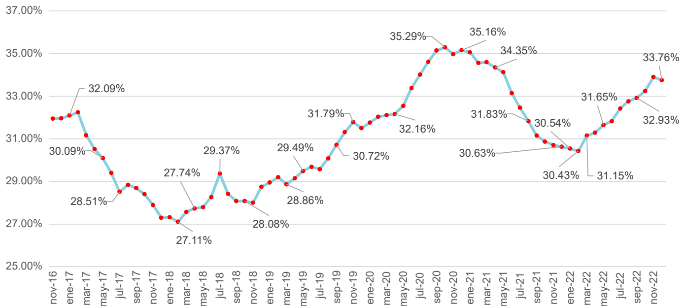
Gráfica 74 - Histórico de porcentaje de pérdidas eléctricas de Honduras 2015-2022
