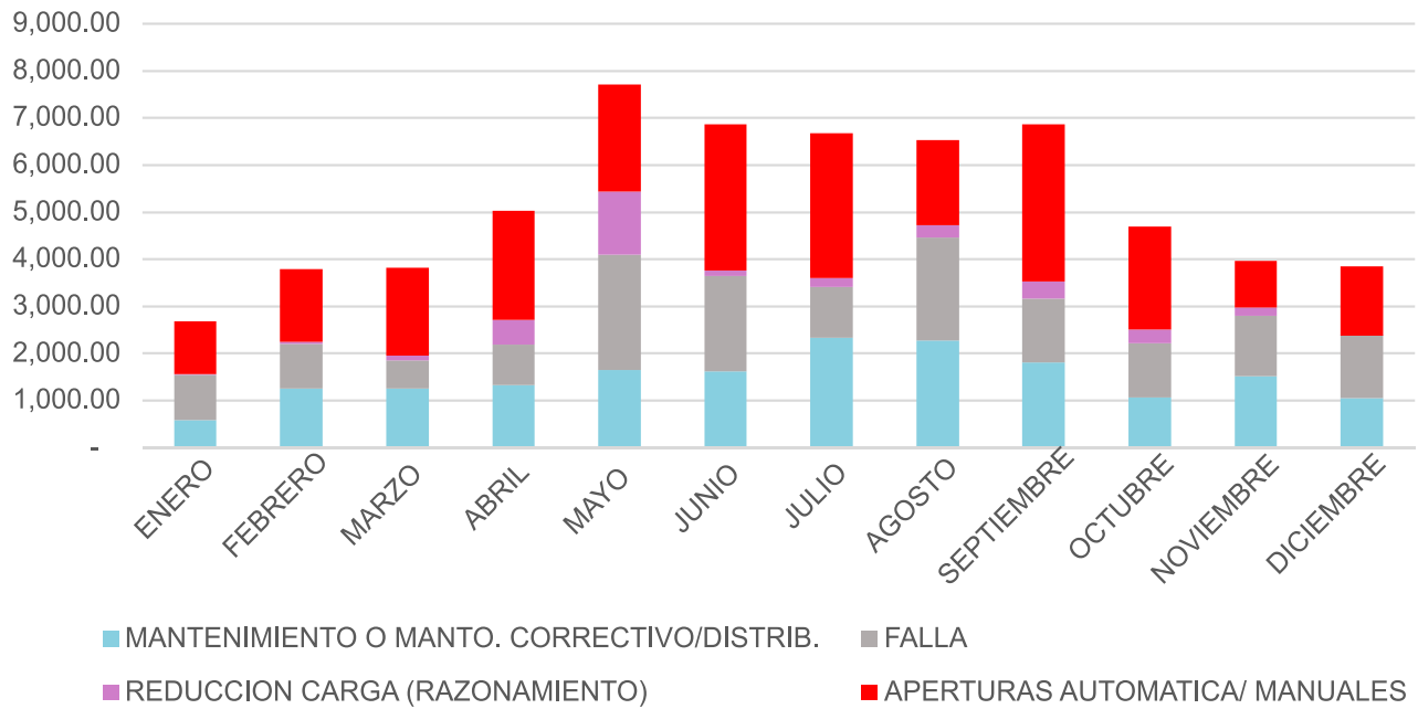
Gráfica 73 - Energía mensual no suministrada en Honduras [MWh] 2022
