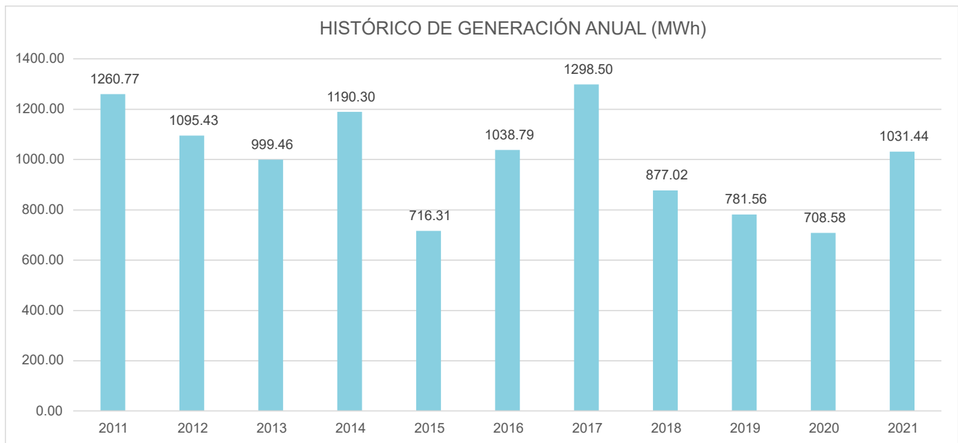
Gráfica 89 - Histórico de generación anual de INELEM [MWh]
