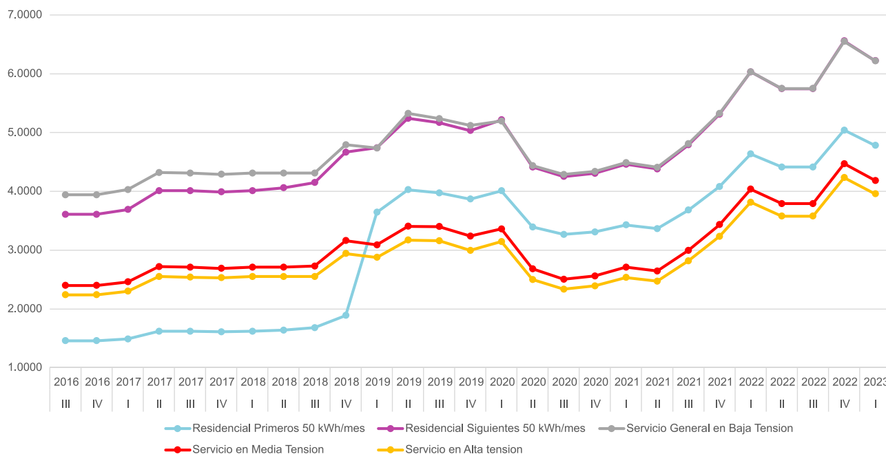
Gráfica 68 - Histórico de tarifa de la energía eléctrica
