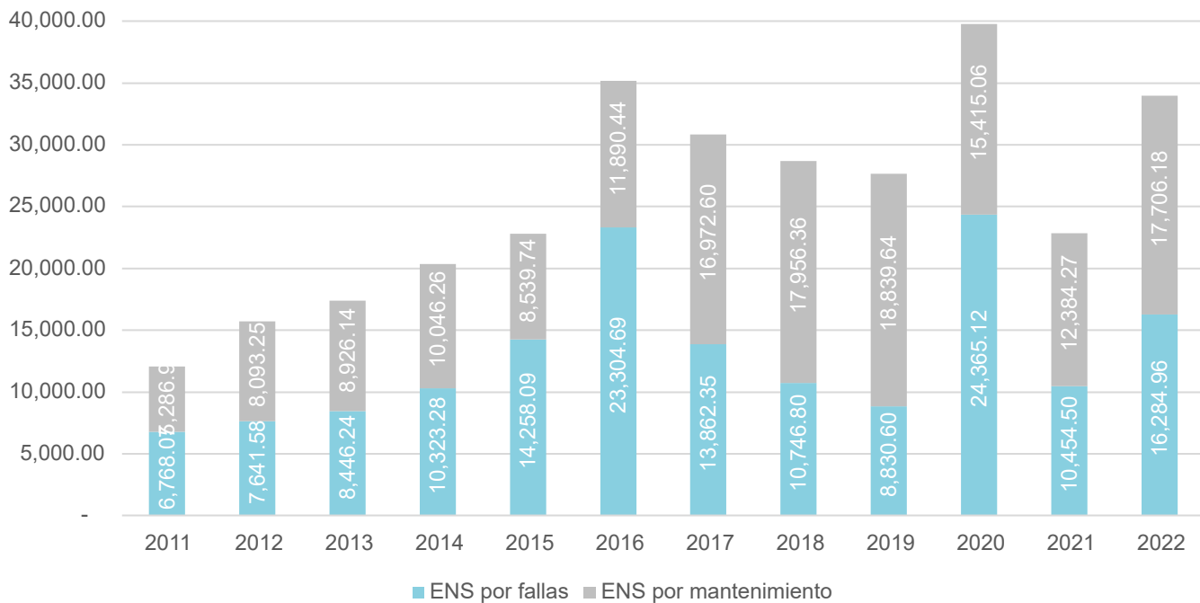
Ilustración 19 - Histórico de energía no suministrada 2011-2022 [MWh]
