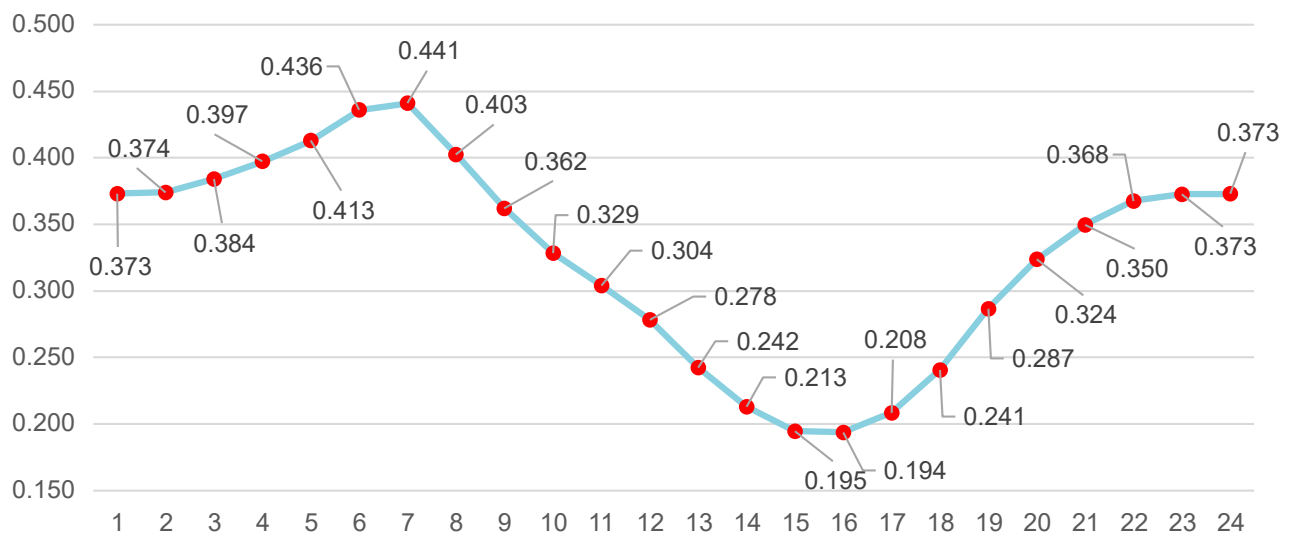
Gráfica 13 - Curva típica de generación eólica en Honduras [p. u.], Base P.U.= 235 MW.
