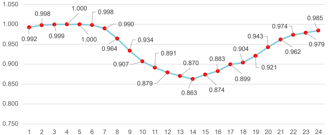
Gráfica 20 - Curva de generación diaria para una planta geotérmica de Honduras [p. u.]
