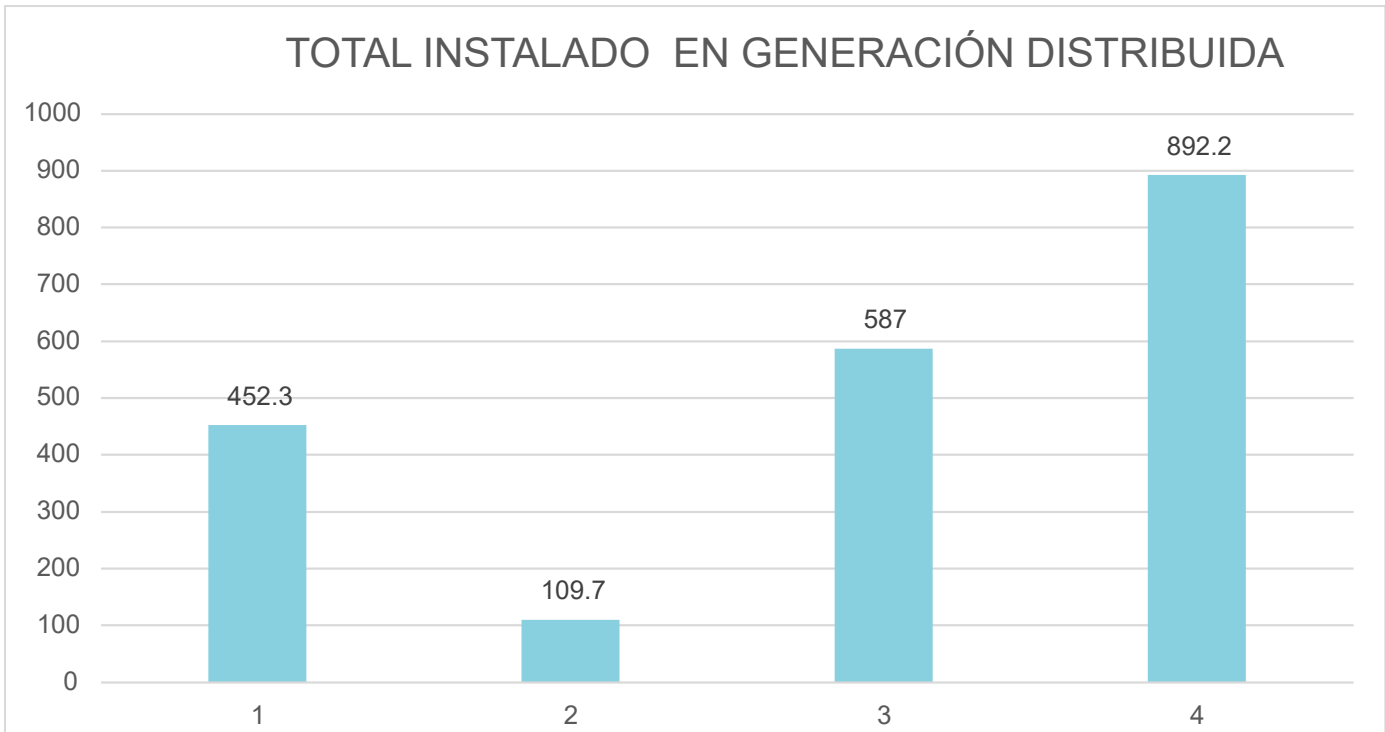
Gráfica 95 - Potencia instalada por regiones de Honduras para generación distribuida [MW]
