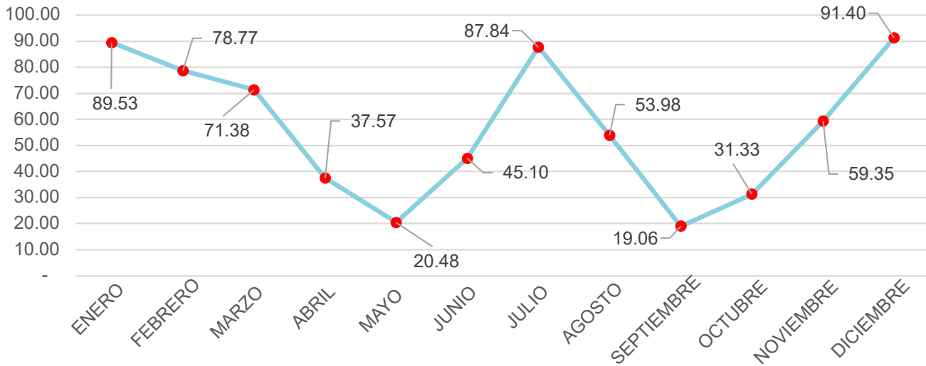
Gráfica 21 - Curva de generación anual para plantas eólicas [GWh]
