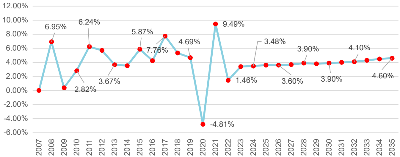
Gráfica 43 - Variación porcentual anual de la proyección de demanda de energía en Honduras
