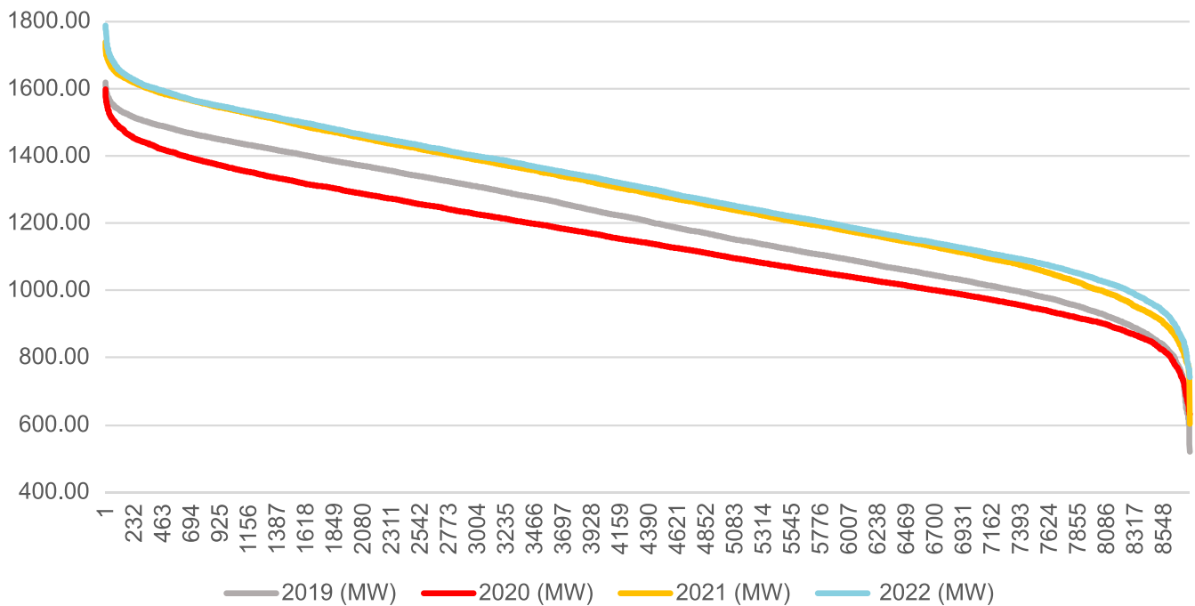
Gráfica 97 - Comparación de curvas de duración de carga 2019, 2020, 2021 y 2022 [MW]
