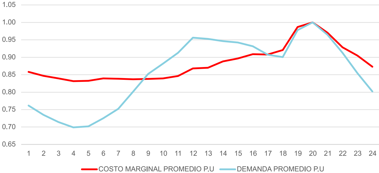
Gráfica 52 - Comparación de tendencias Por Unidad (P.U.) - Costo Marginal vrs Demanda
