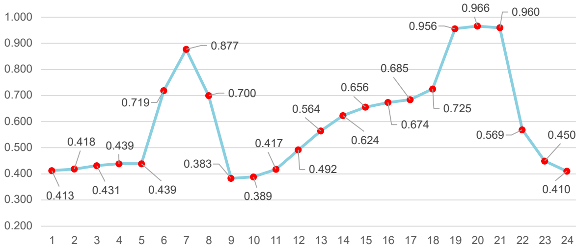
Gráfica 18 - Curva típica de generación típica de La Vegona [p. u.]
