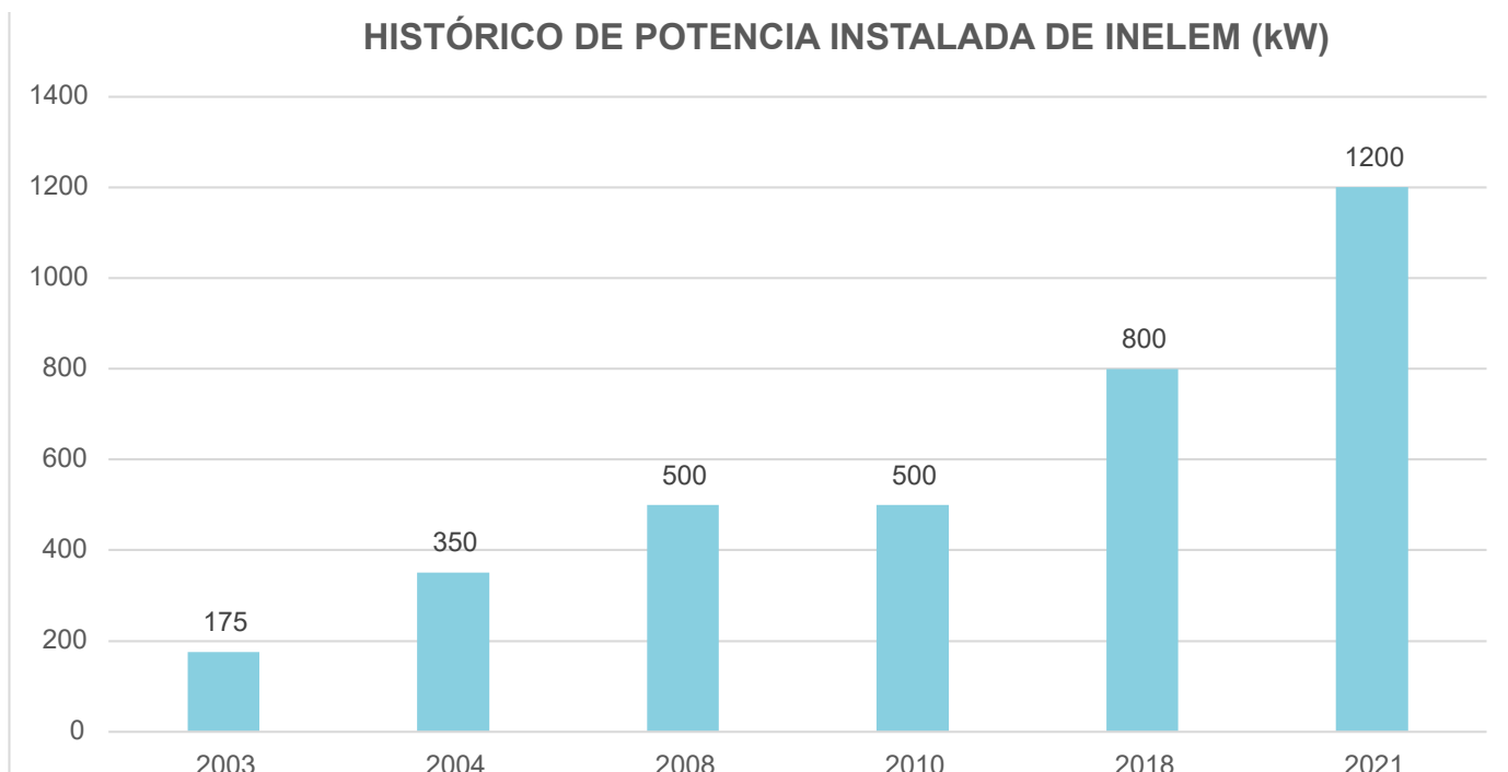
Gráfica 90 - Histórico de potencia instalada de INELEM 2003-2018 [kWh]
