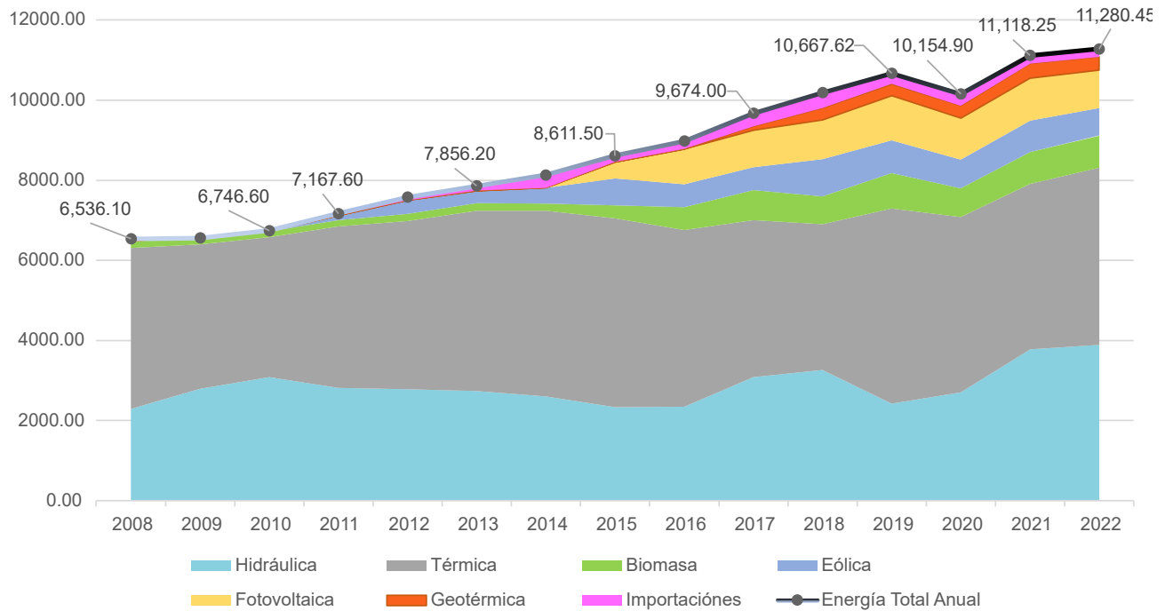
Gráfica 10 - Histórico de generación acumulada en Honduras (GWh) 2008-2022
