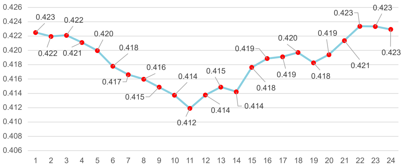
Gráfica 19 - Curva de generación diaria para plantas de biomasa instaladas en Honduras [p. u.]
