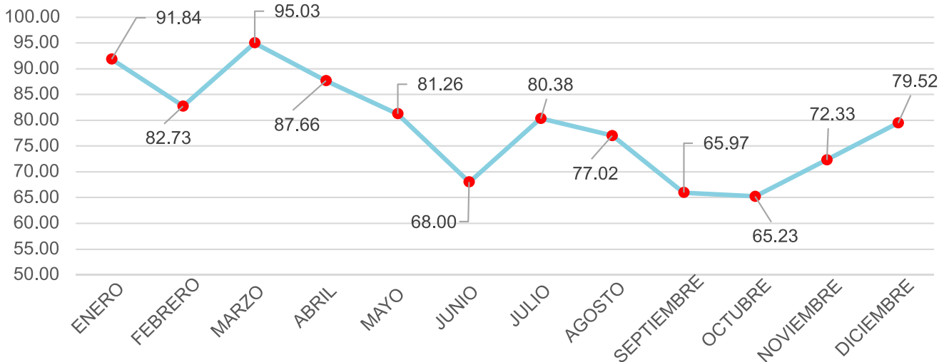
Gráfica 22 - Curva de generación anual para plantas solares [GWh]
