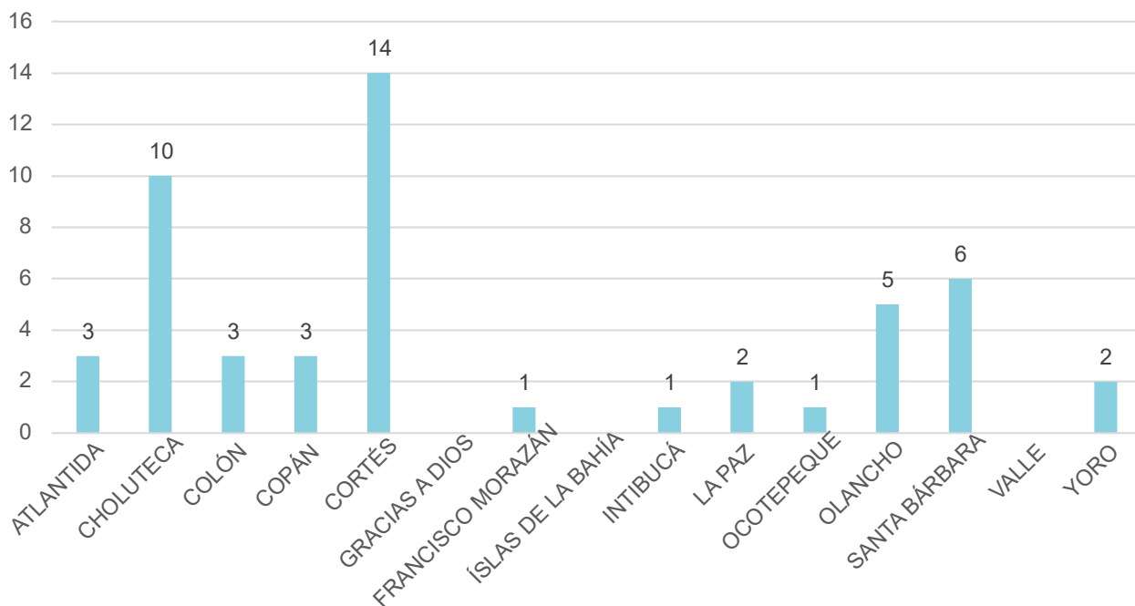
Gráfica 31 - Número de centrales hidroeléctricas por departamento 2022
