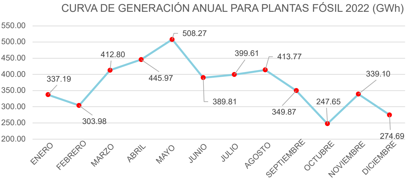
Gráfica 24 - Curva de generación anual de plantas térmicas a base combustibles fósiles [GWh]
