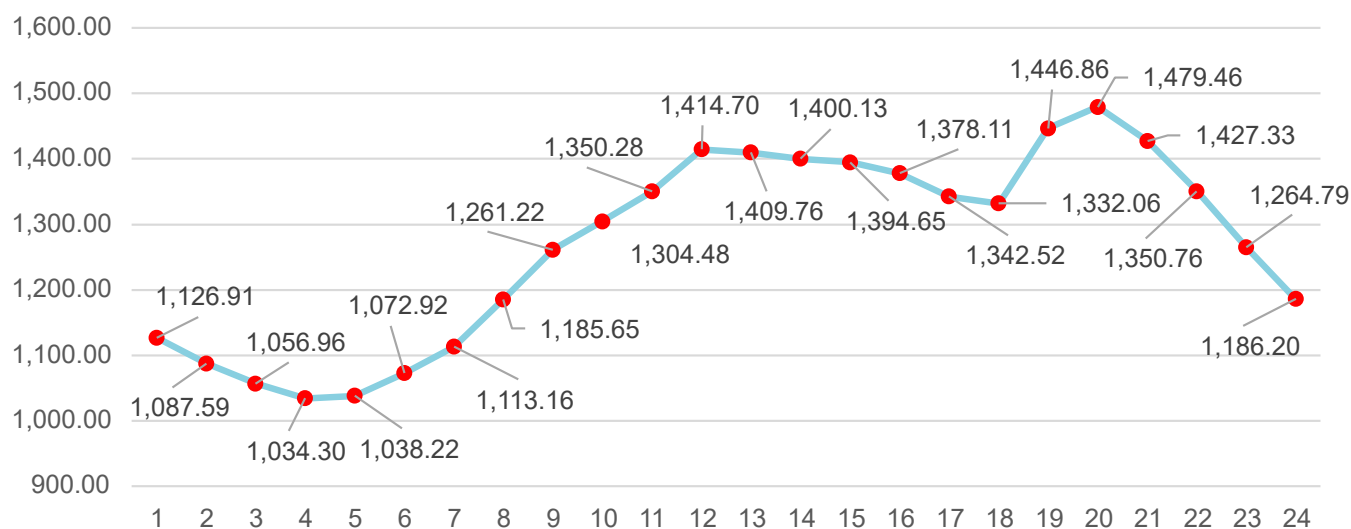
Gráfica 36 - Demanda eléctrica diaria promedio 2022 en Honduras [MW]
