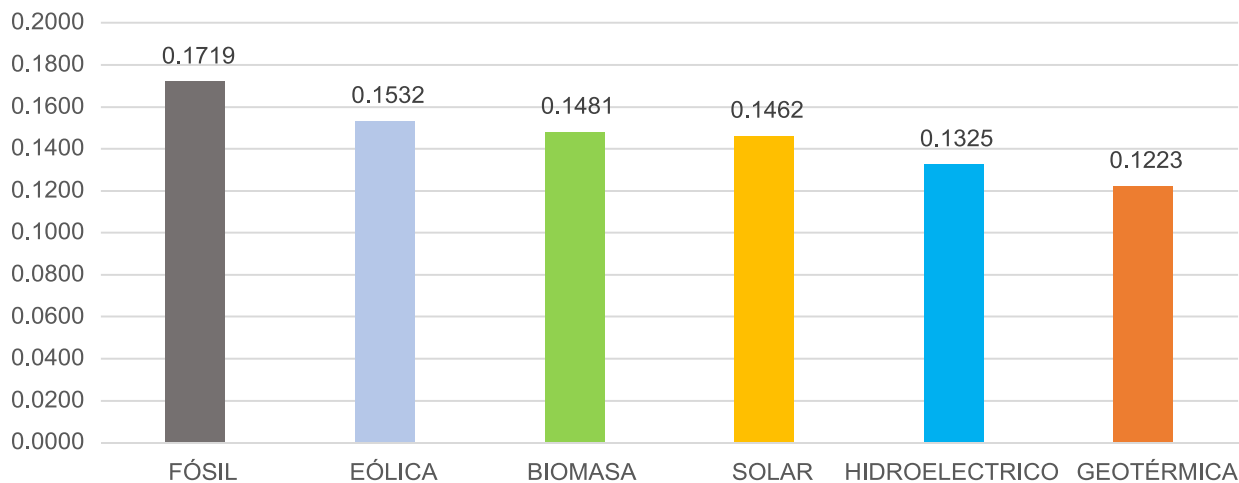
Gráfica 44 - Precio monómico por tecnología de generación [USD/kWh]
