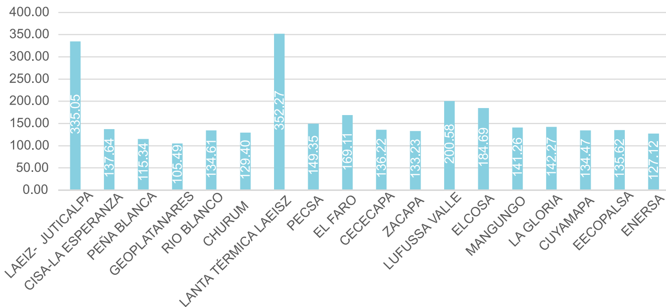
Gráfica 50 - Precios promedio de las plantas del Mercado de Oportunidad Nacional [USD/MWh]
