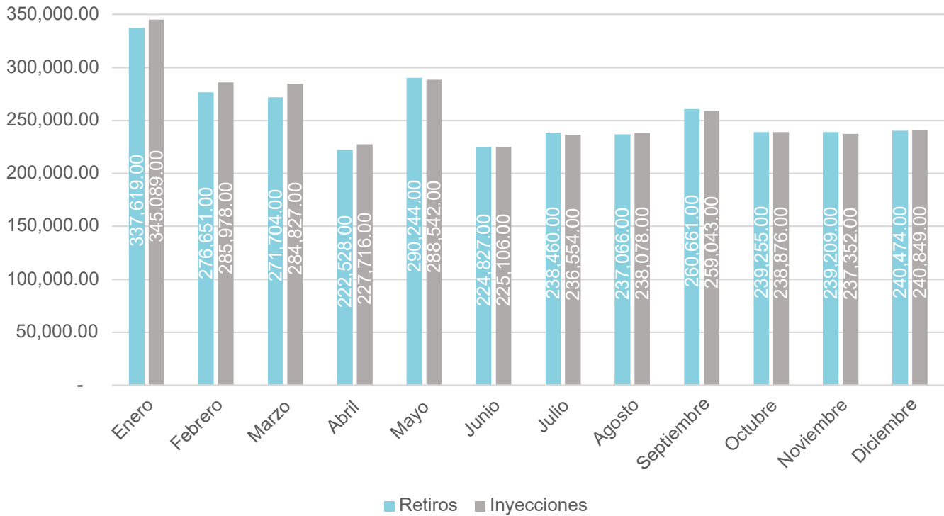
Gráfica 80 - Inyecciones y retiros totales en el MER 2022 [MWh]
