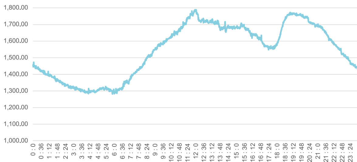
Gráfica 37 - Curva de demanda del día con la demanda máxima del año 2022 en Honduras
