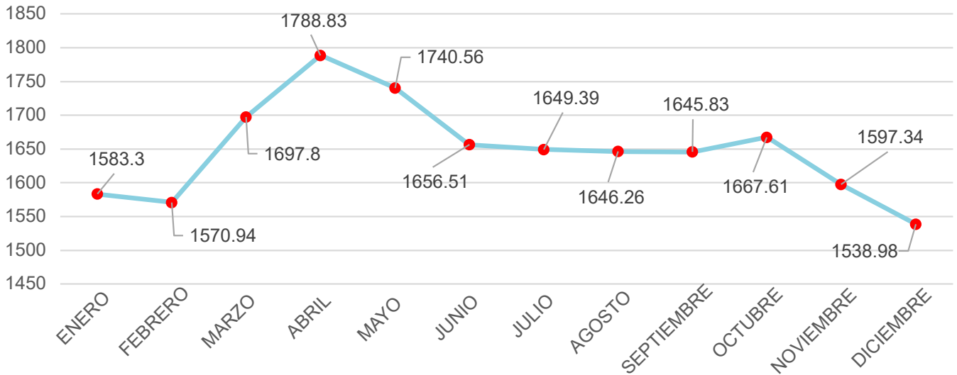
Gráfica 39 - Demanda máxima mensual en Honduras 2022 [MW]
