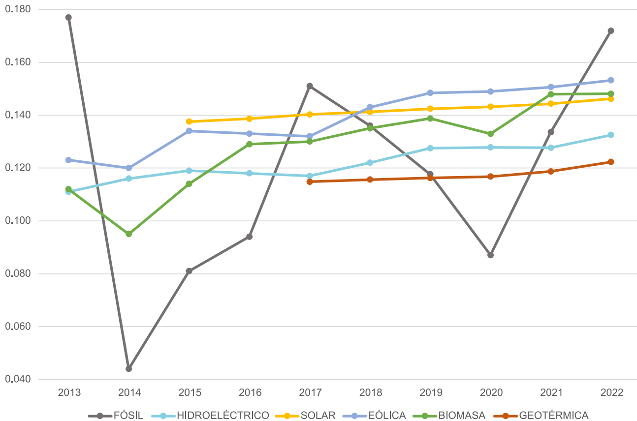
Gráfica 47 - Precios históricos de la energía eléctrica por tecnología [USD/kWh]
