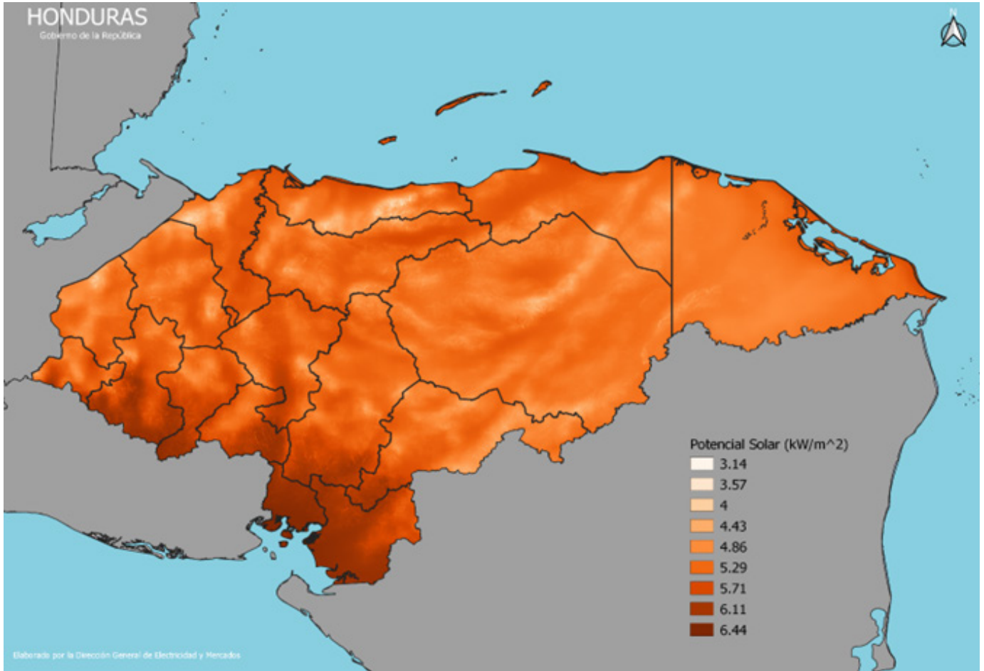
Ilustración 11 – Mapa de potencial solar de Honduras
