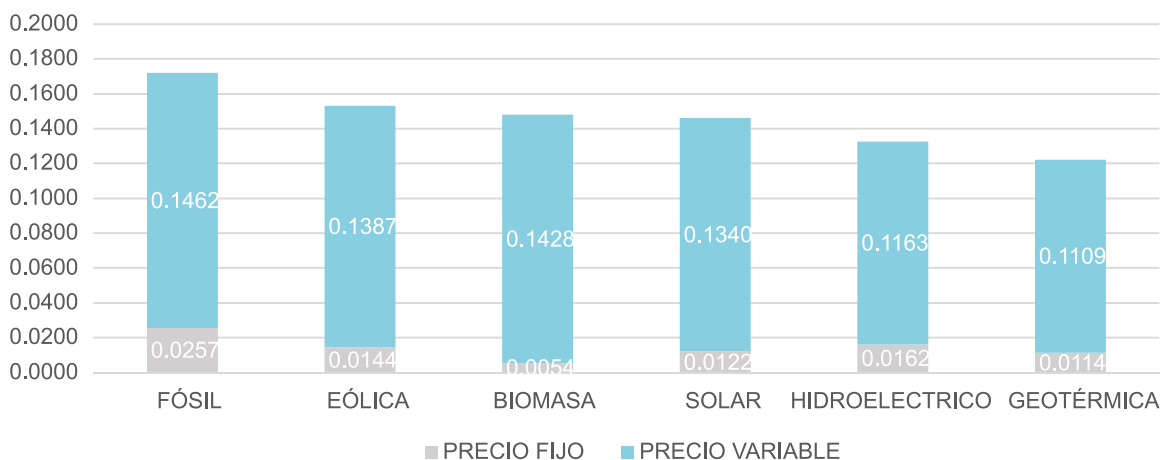
Gráfica 45 - Precios/cargos fijos y variables por tecnología [USD/kWh]
