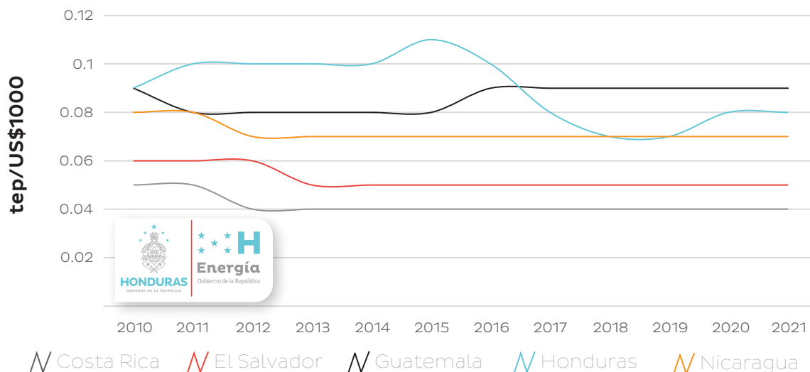
Figura 80. Indicador de intensidad energética en Centroamérica 2010 - 2021
