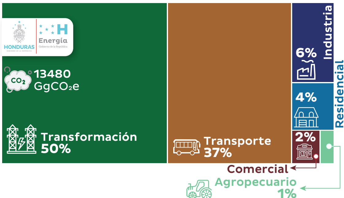
Figura 75. Emisiones de gases de efecto invernadero según sector de consumo 2022
