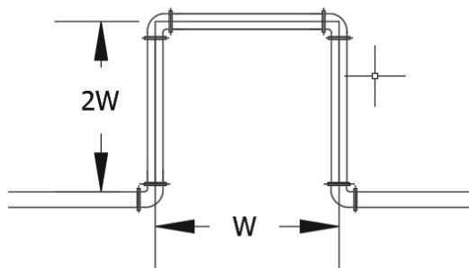
Figura No.7 "Loops" de expansión
