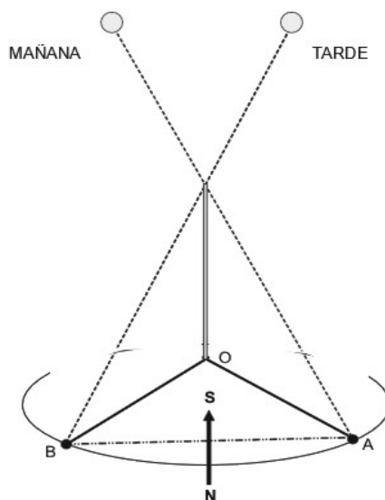
Figura No.15 Determinación del sur geográfico
