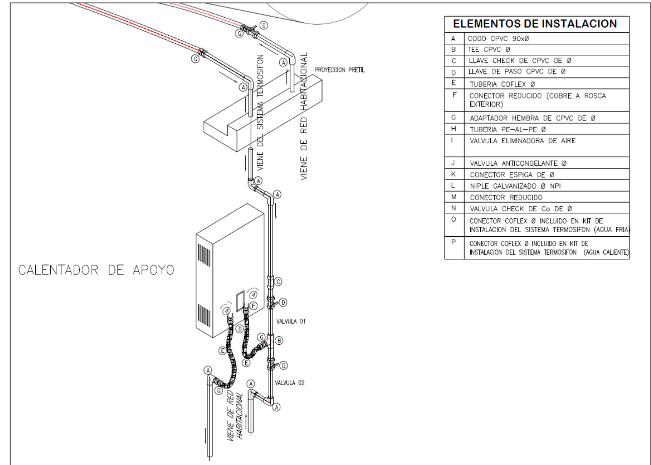
Figura No.13 Conexión de sistema solar tipo termosifón con respaldo
