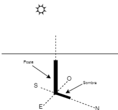
Figura No.14. Determinación del sur geográfico mediante proyecto de sombra en hora de culminación solar
