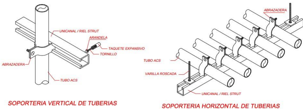
Figura No.6 Soportaría de tuberías
